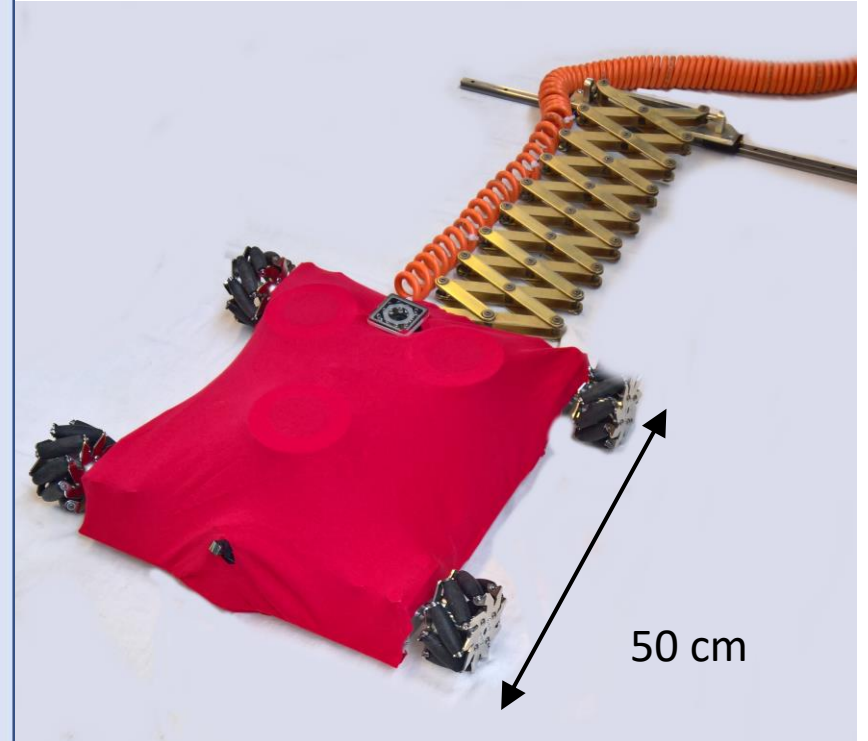
Automatisches Laden von Elektroautos z.B. in Parkhäusern mit dem Charge-Crawler
